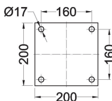
Construção do Cabeçote Head Construction / Construcción del cabezal
