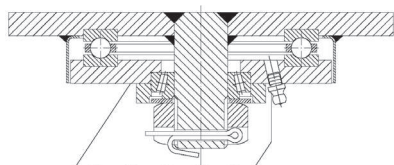
Construção do Cabeçote Head Construction / Construcción del cabezal
