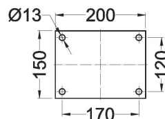
Placa de Fixação para MPAX 123/153 Fitting plate for MPAX 123/153 Placa de fijación para MPAX 123/153
