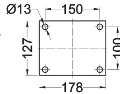
Placa de Fixação para MPAX 103 Fitting plate for MPAX 103 Placa de fijación para MPAX 103
